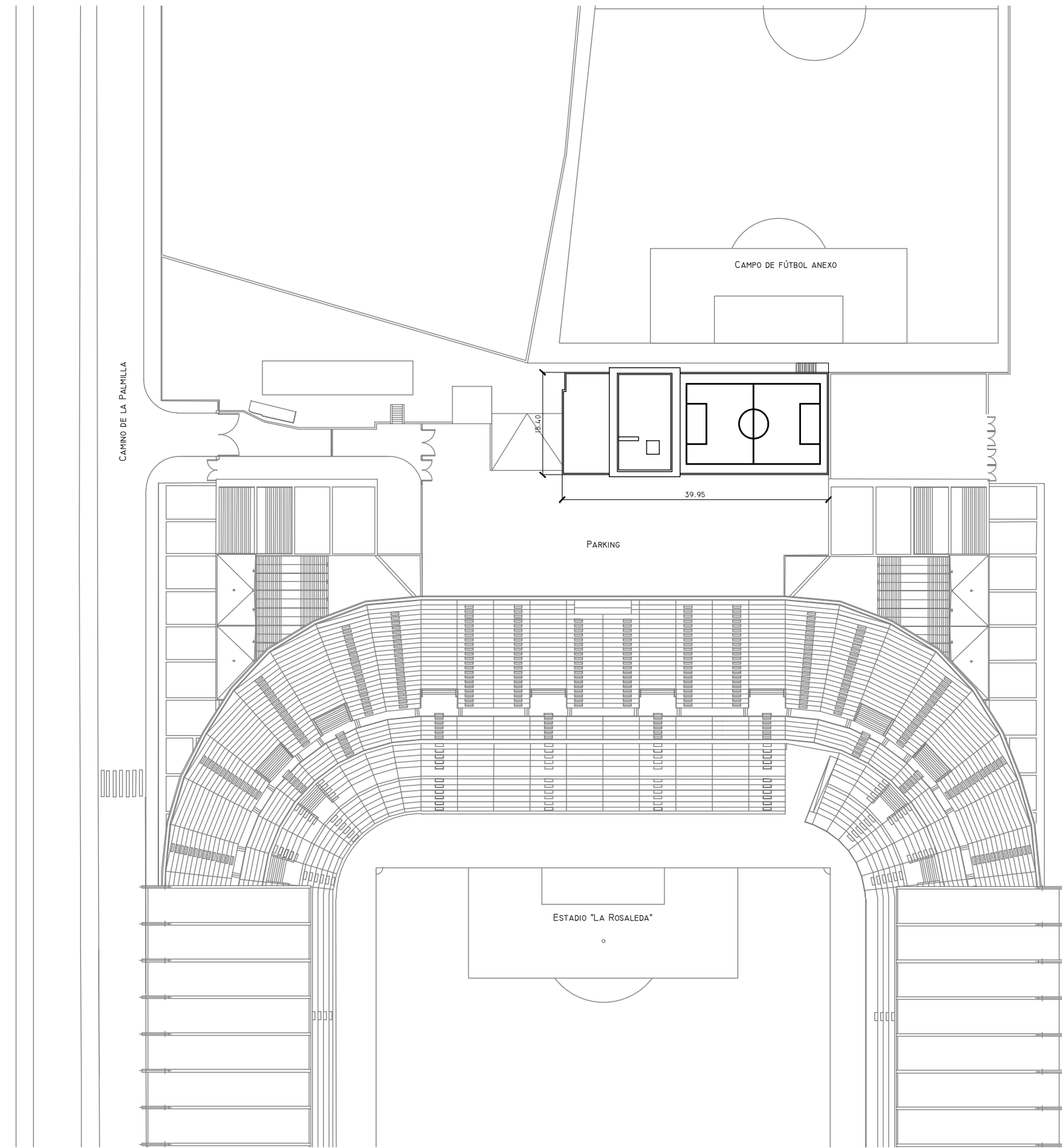
EMPLAZAMIENTO. UBICACIÓN NUEVO EDIFICIO ESCALA 1:750
